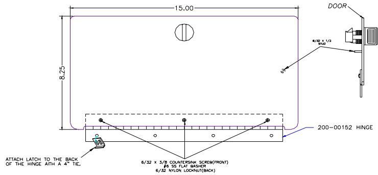
205-00185-A & 205-00186-A GLOVE BOX DOOR
