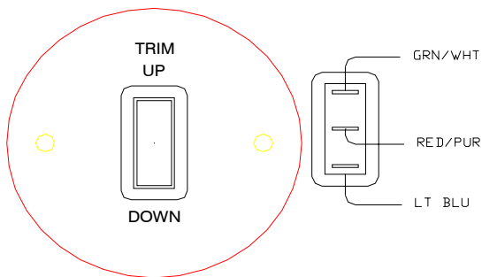
205-00205-A SE TRANSOM TRIM PANEL (VOLVO)
