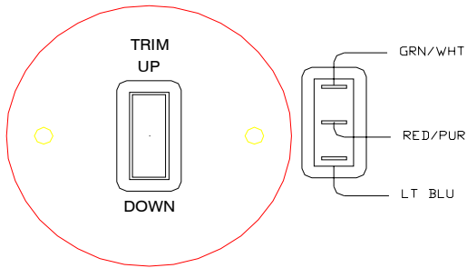
205-00205-A SE TRANSOM TRIM PANEL (VOLVO)
