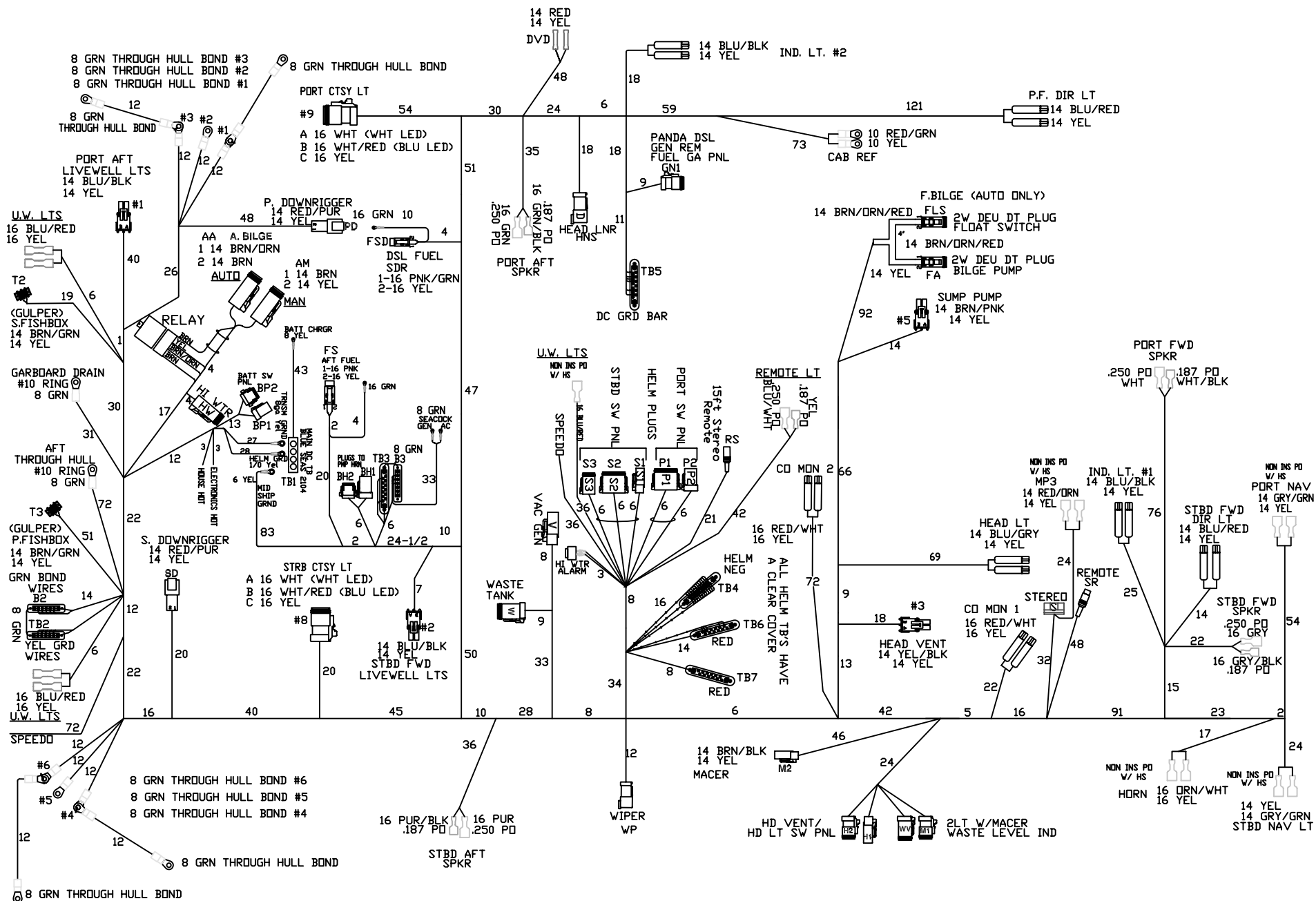
Robalo 305
