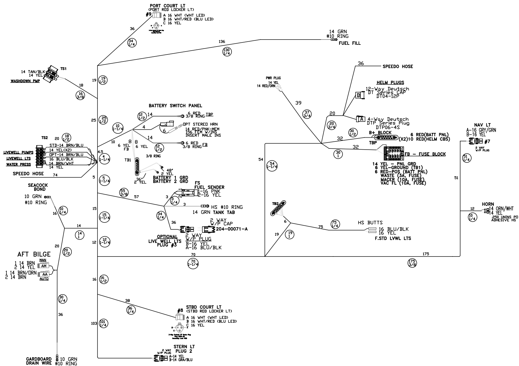
Robalo 220
