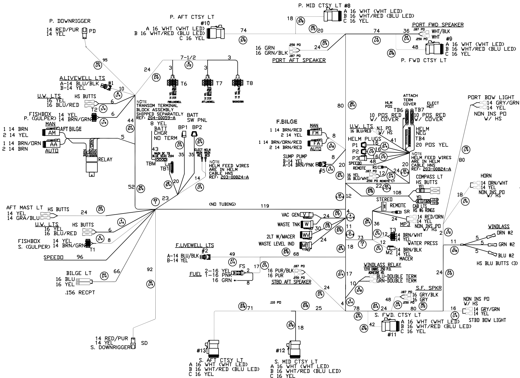
Robalo 300
